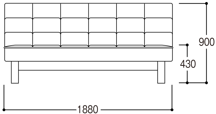
正面图
