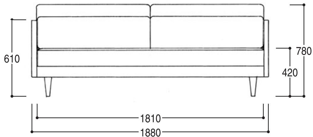
正面图 3P
