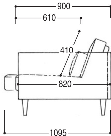
侧面图 3P
