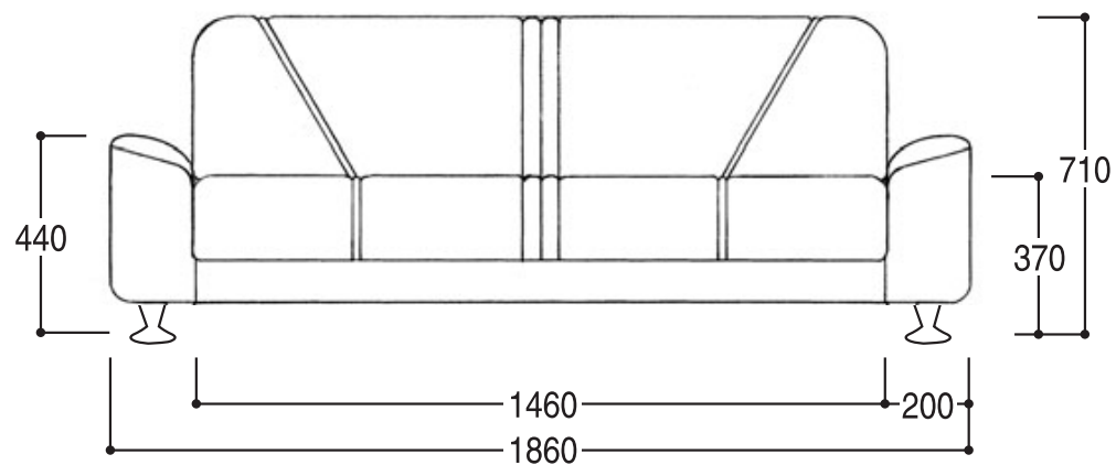
正面図
