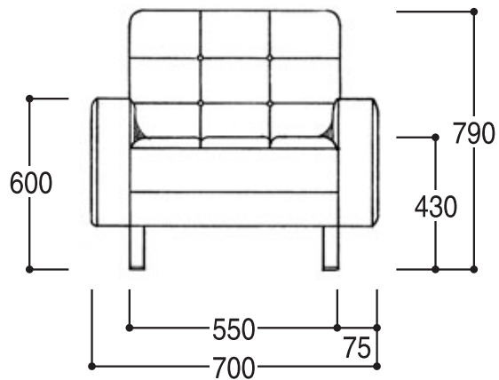
正面図 1P
