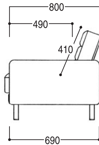
側面図 1P
