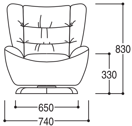
正面図 1P
