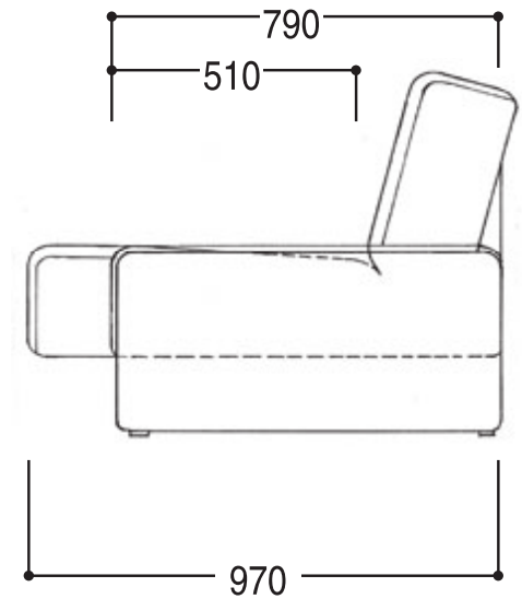
侧面图
