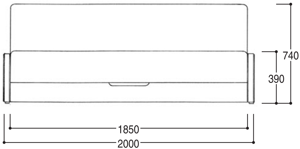
正面图
