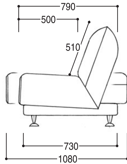
側面図 ハイバック
