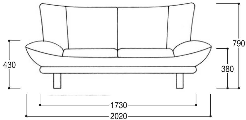
正面図
