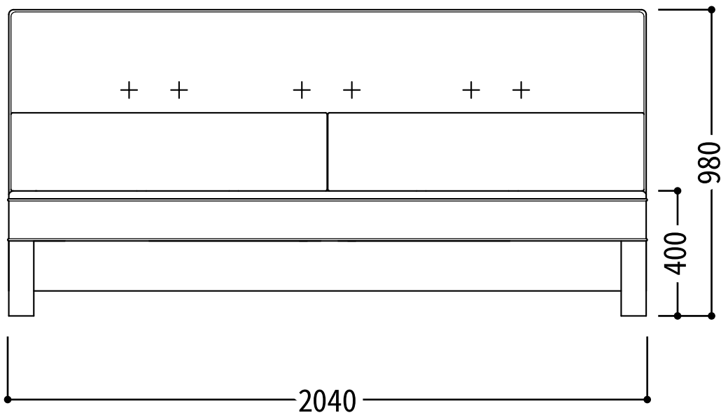
正面图
